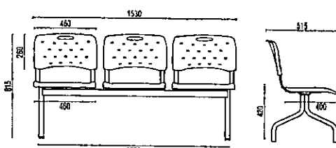
35010 Longarina Larguras sem Braço: 2L - 1026mm 3L - 1530mm 4L - 2052mm 5L - 2578mm
